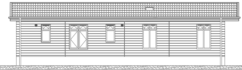
Elevation B
